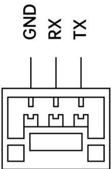
UART
